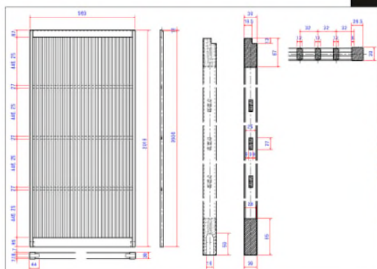
建具図面一例
