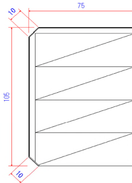
＜床框面皮断面図＞
