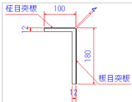
玄関リフォーム 上り框断面図
